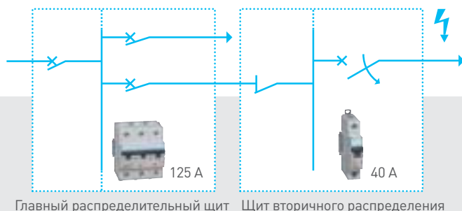
Главный распределительный щит Щит вторичного распределения
